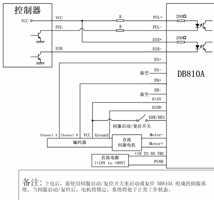
图 8 DB810A 驱动器与 DCM5xxxx 系列电机的接线图
