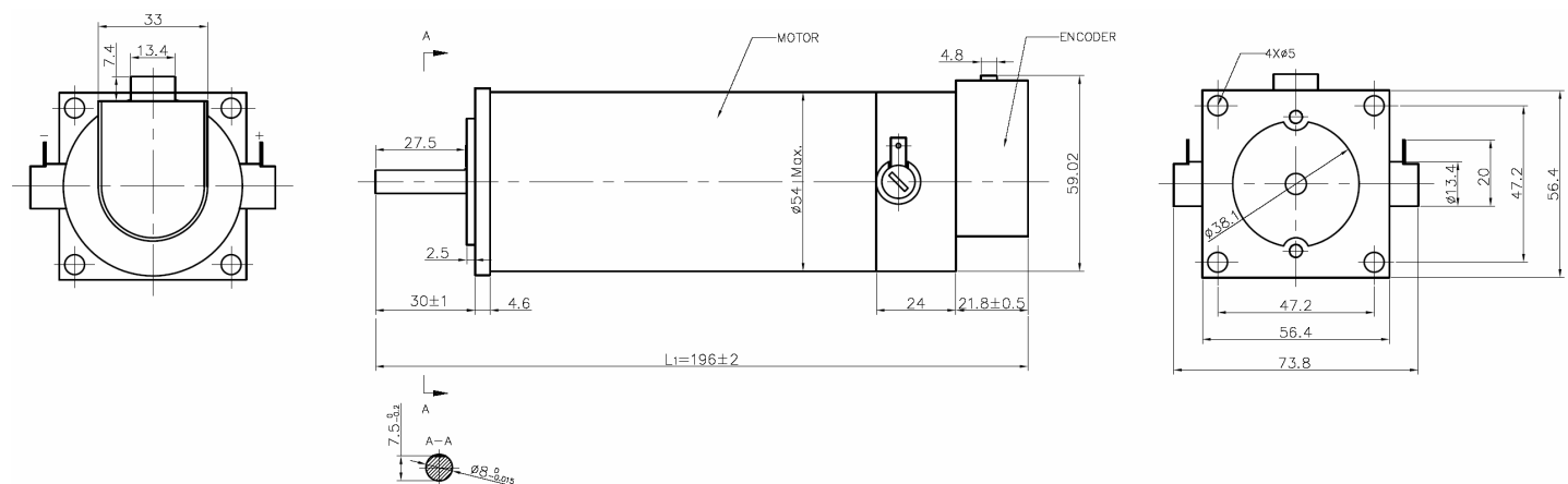
图 3 DCM57207 电机加编码器尺寸图
